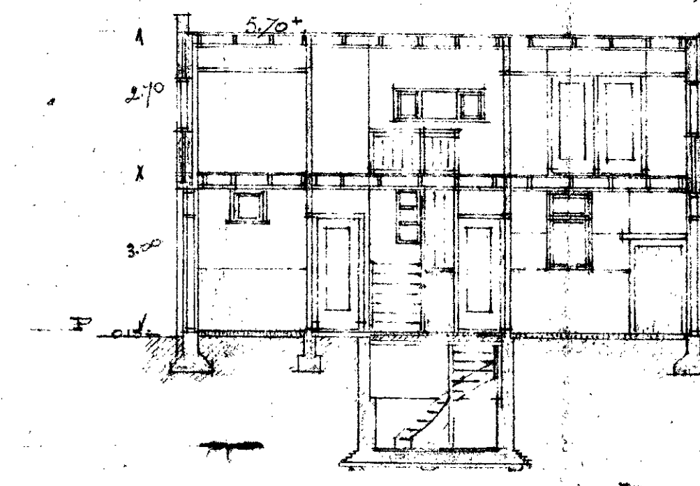
DOORSNEDEN A-D.
