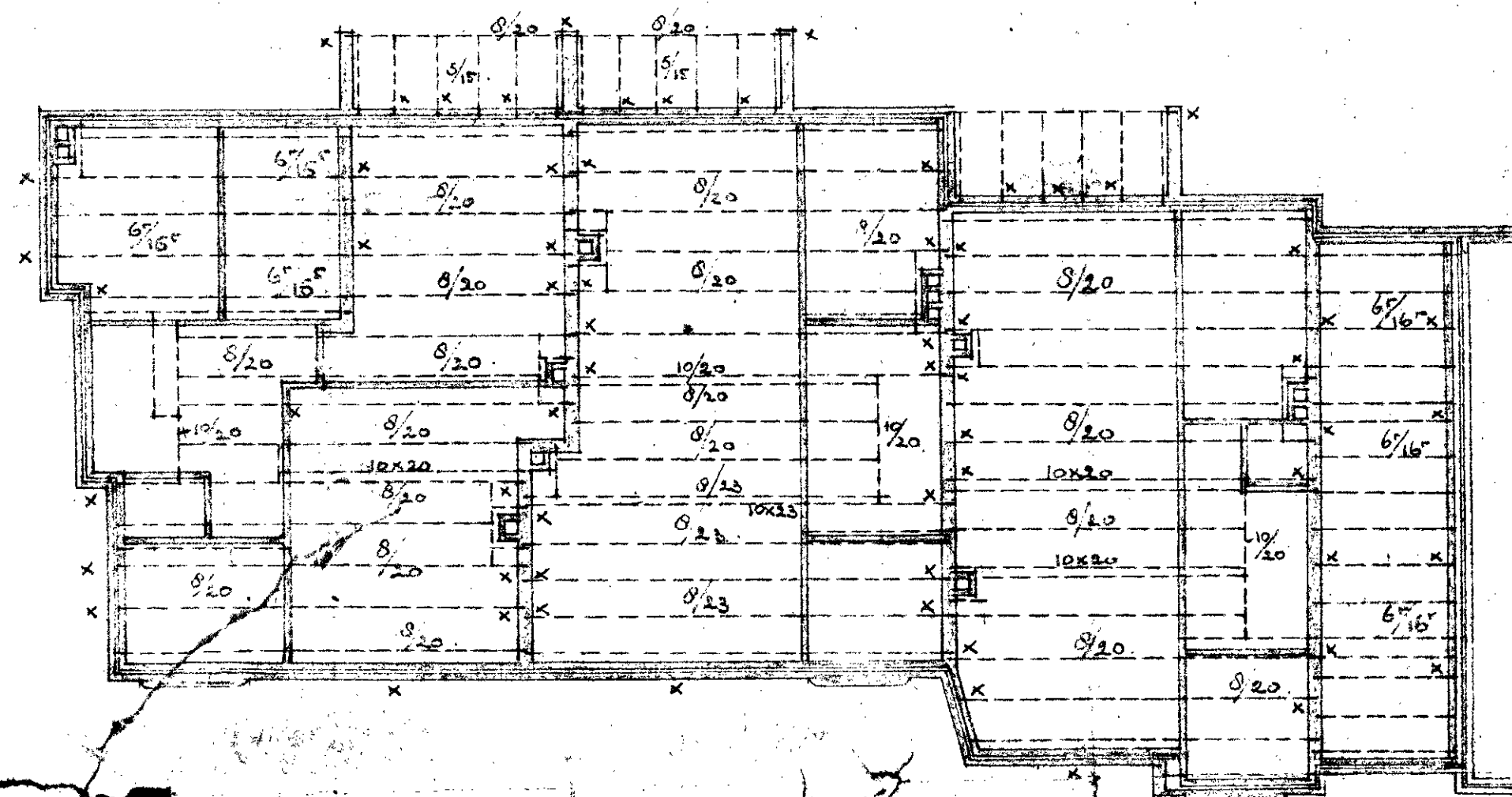
VERDIEPING-BALKLAAG.
