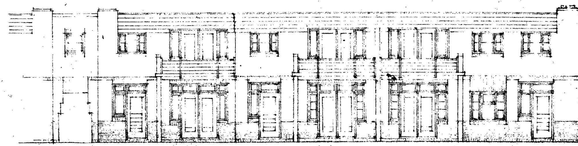
ACHTERGEVEL.
