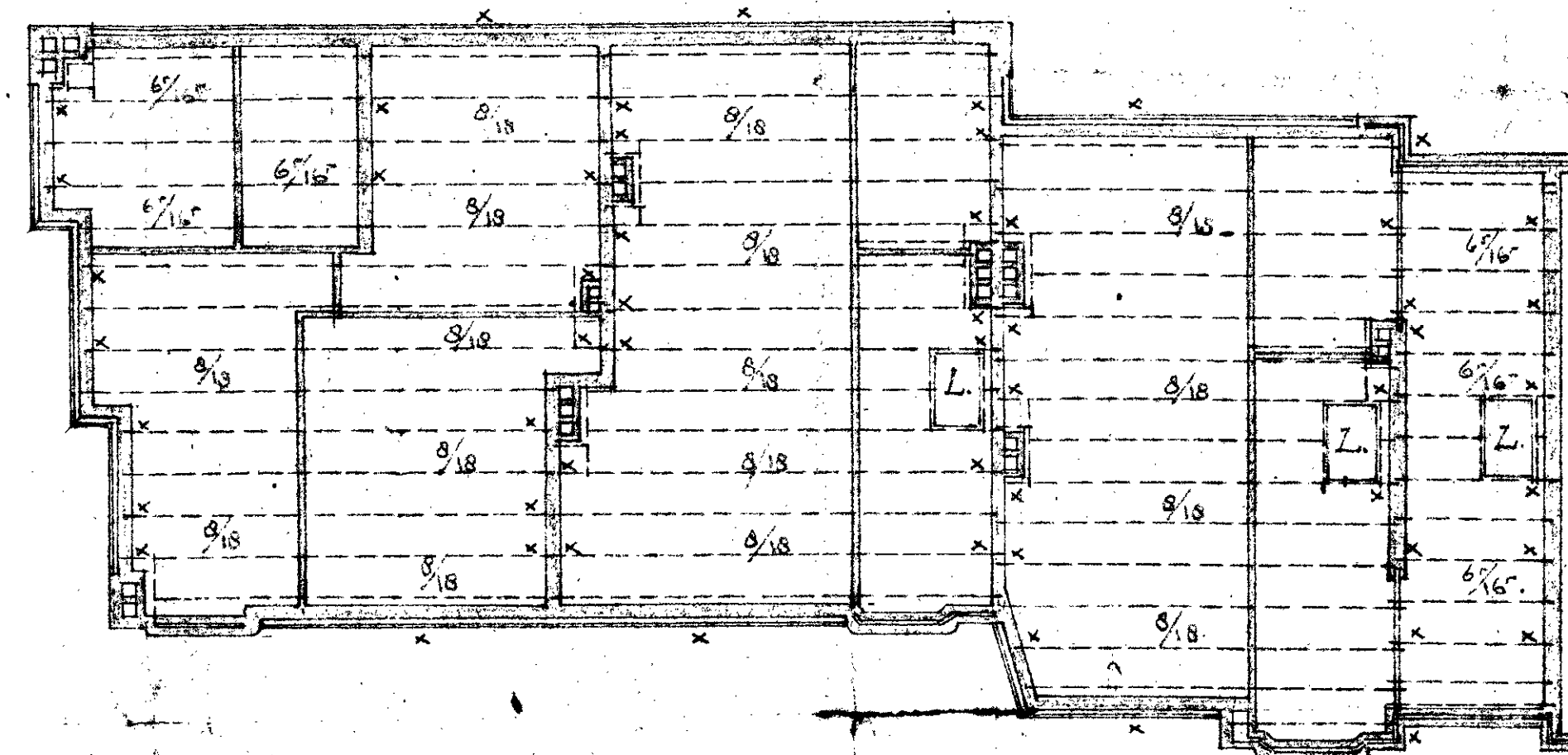
PLAT-BALKLAAG.
