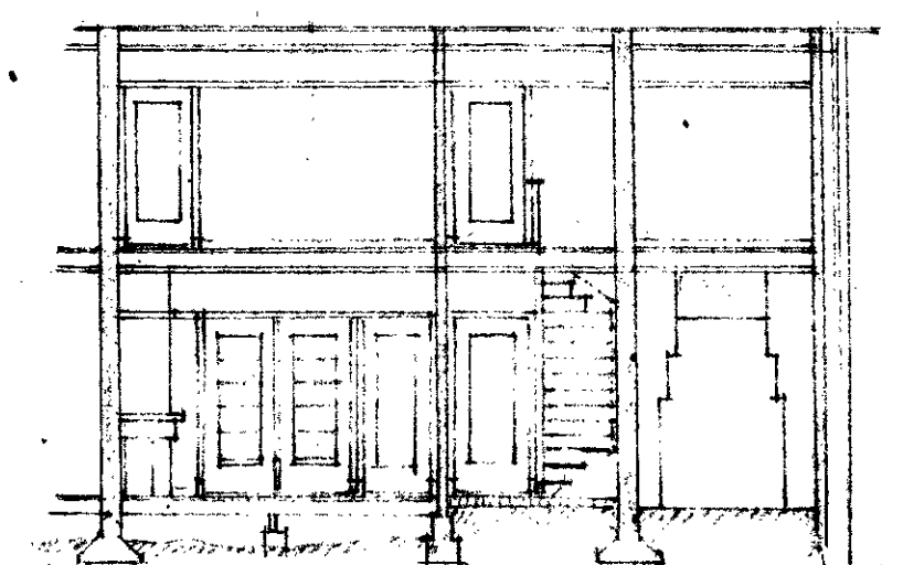
DOORSNEDEN C-D.
