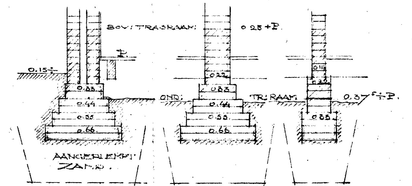
DOORSNEDEN OVER FUNDITEERINGEN SCHAAL 1:20.
