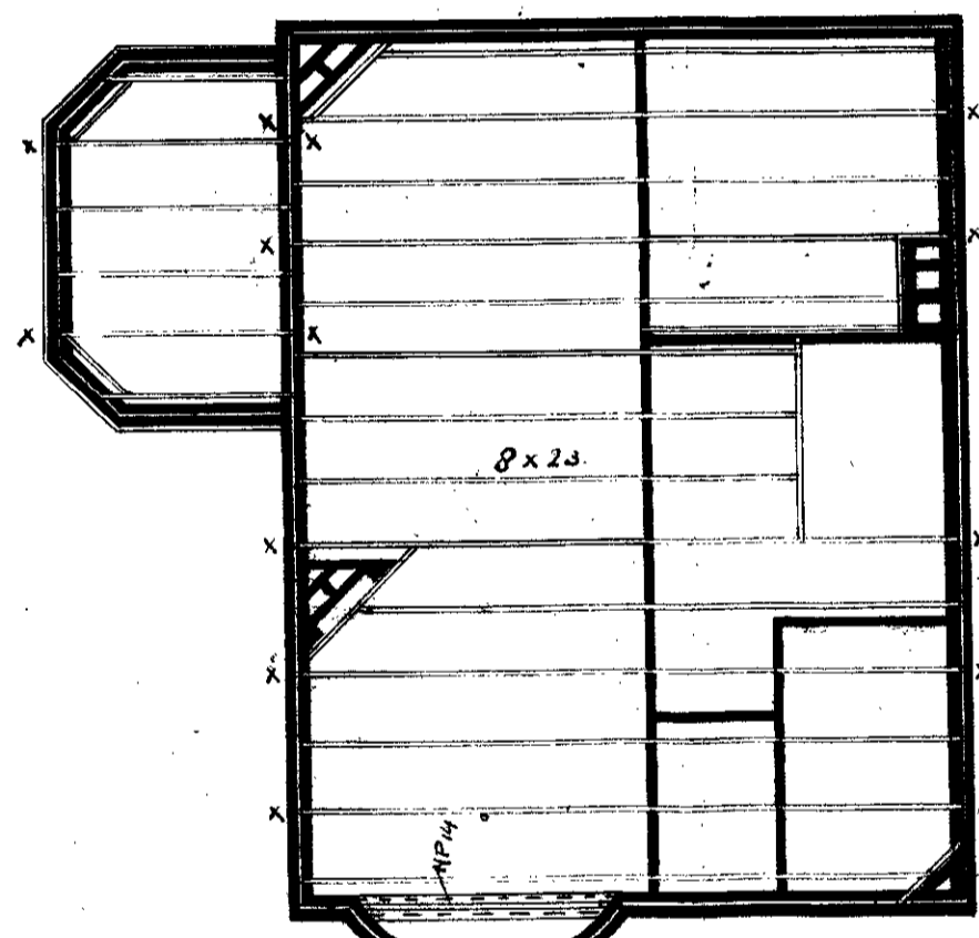
1 ste Daklaag
