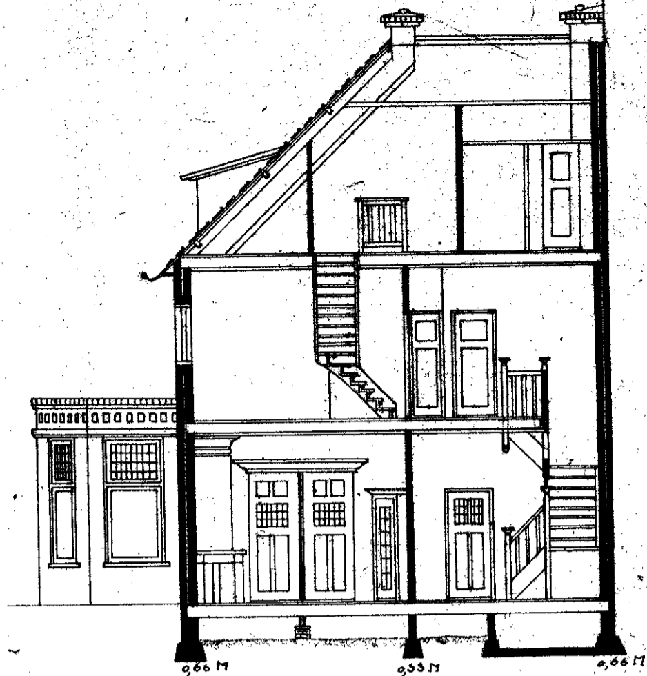
Doorsnede A-B
