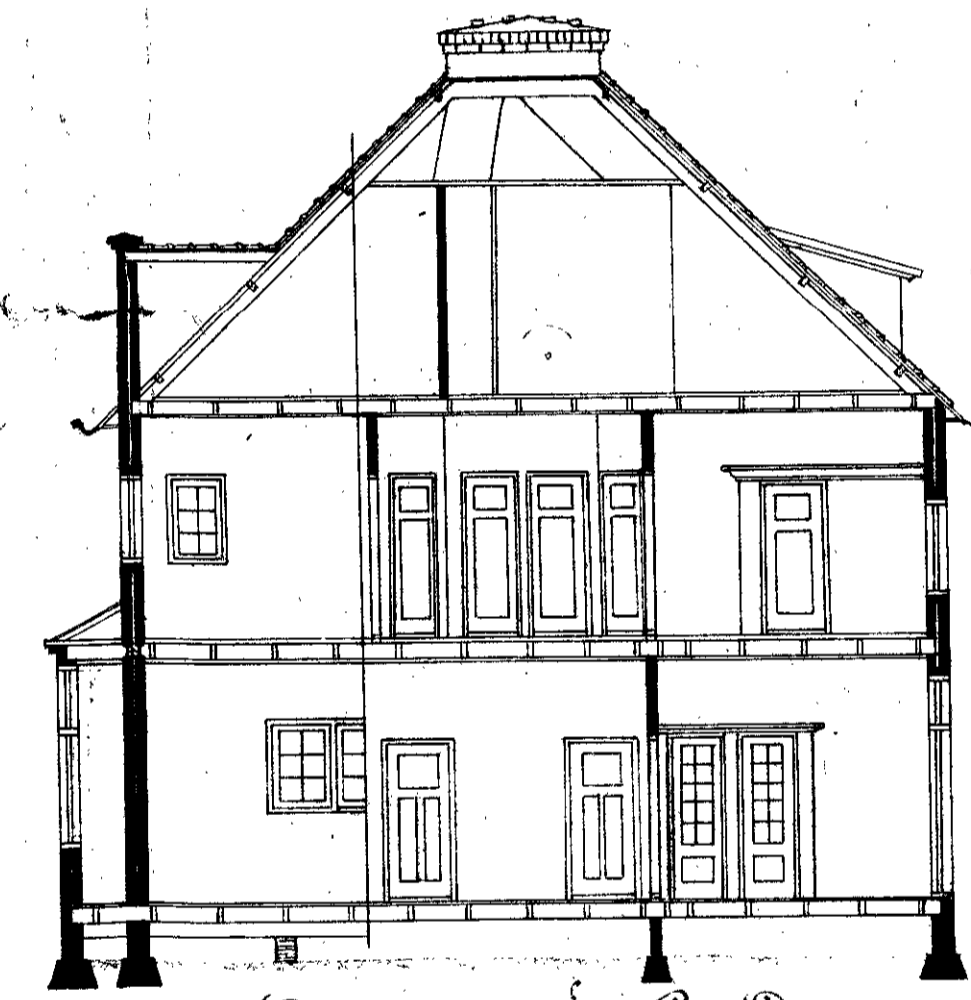
Doorsnede C-D
