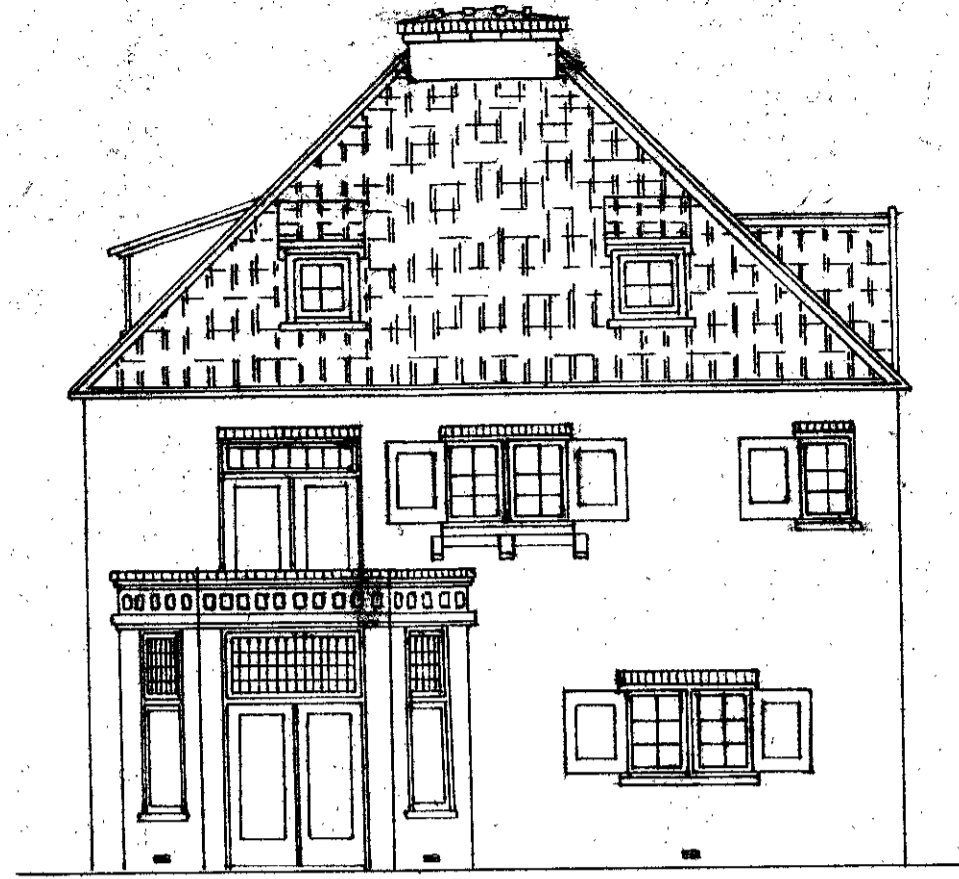
Zijgevel
