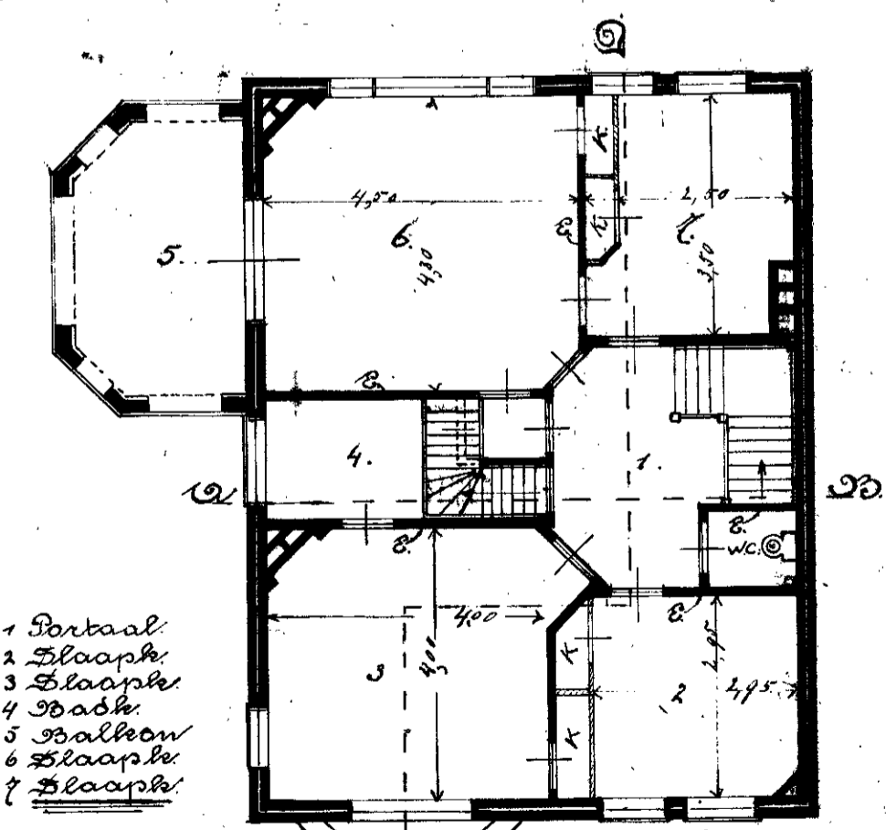
1 ste Verdieping
