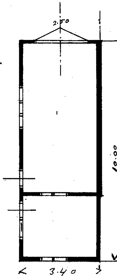
BESTAND PLATTEGROND
