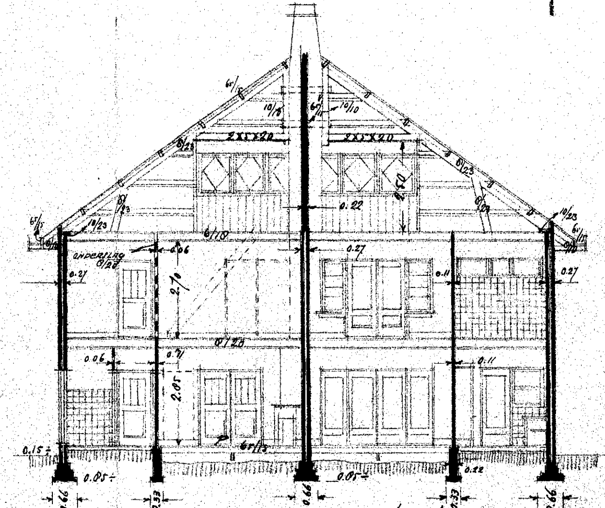
VOORCNEVE A-B
