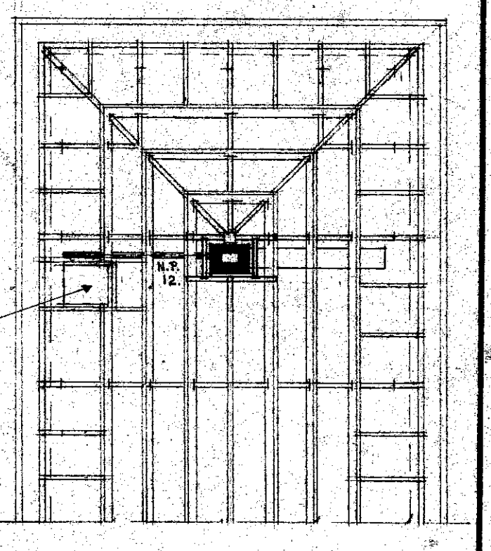
GEDEELTE KAPPLAN (boven voormalige accuruimte)
