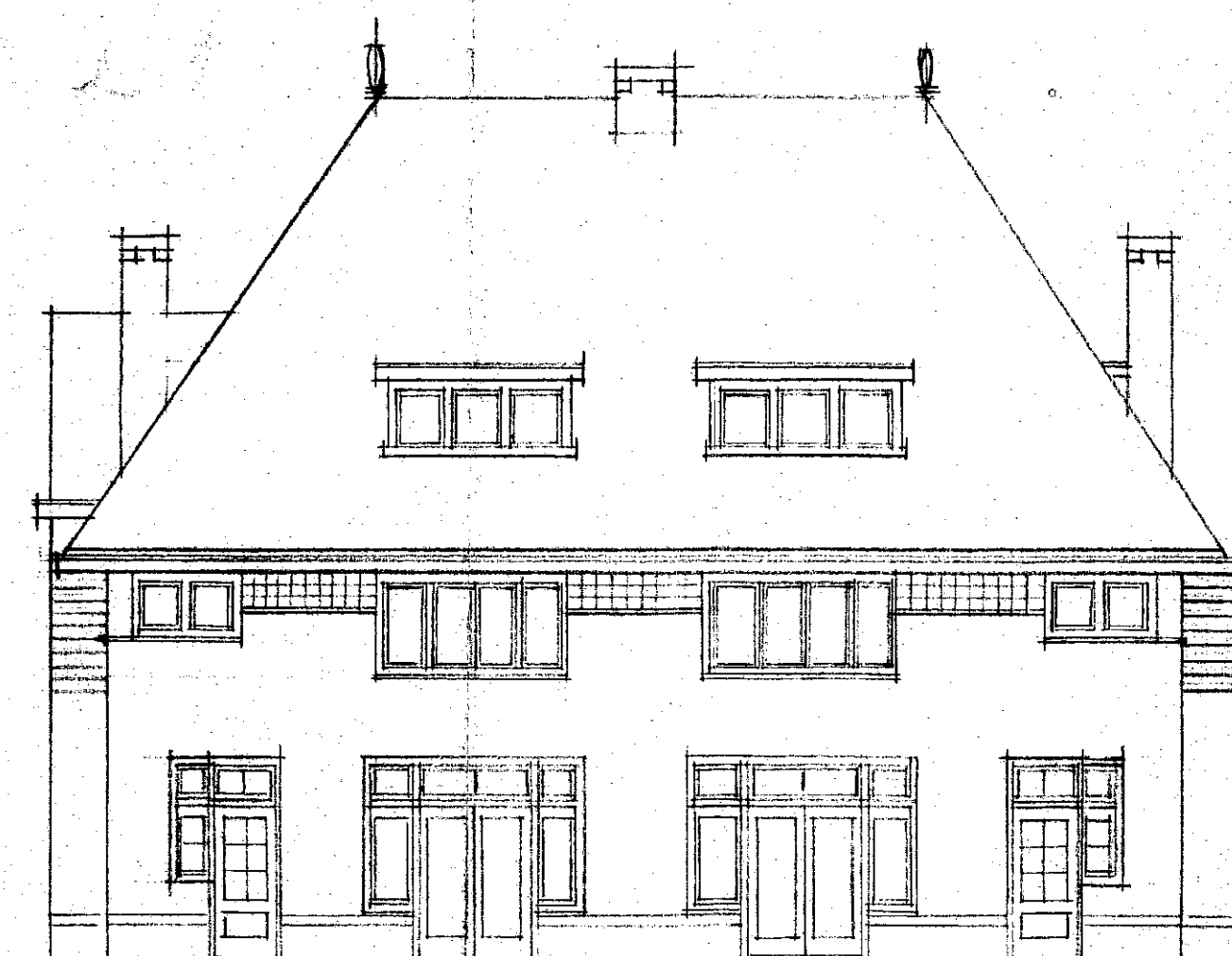
ACHTERGEVEL
