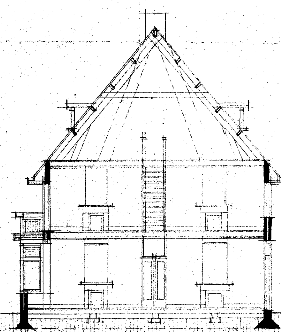
DOORSNEDEN C-D
