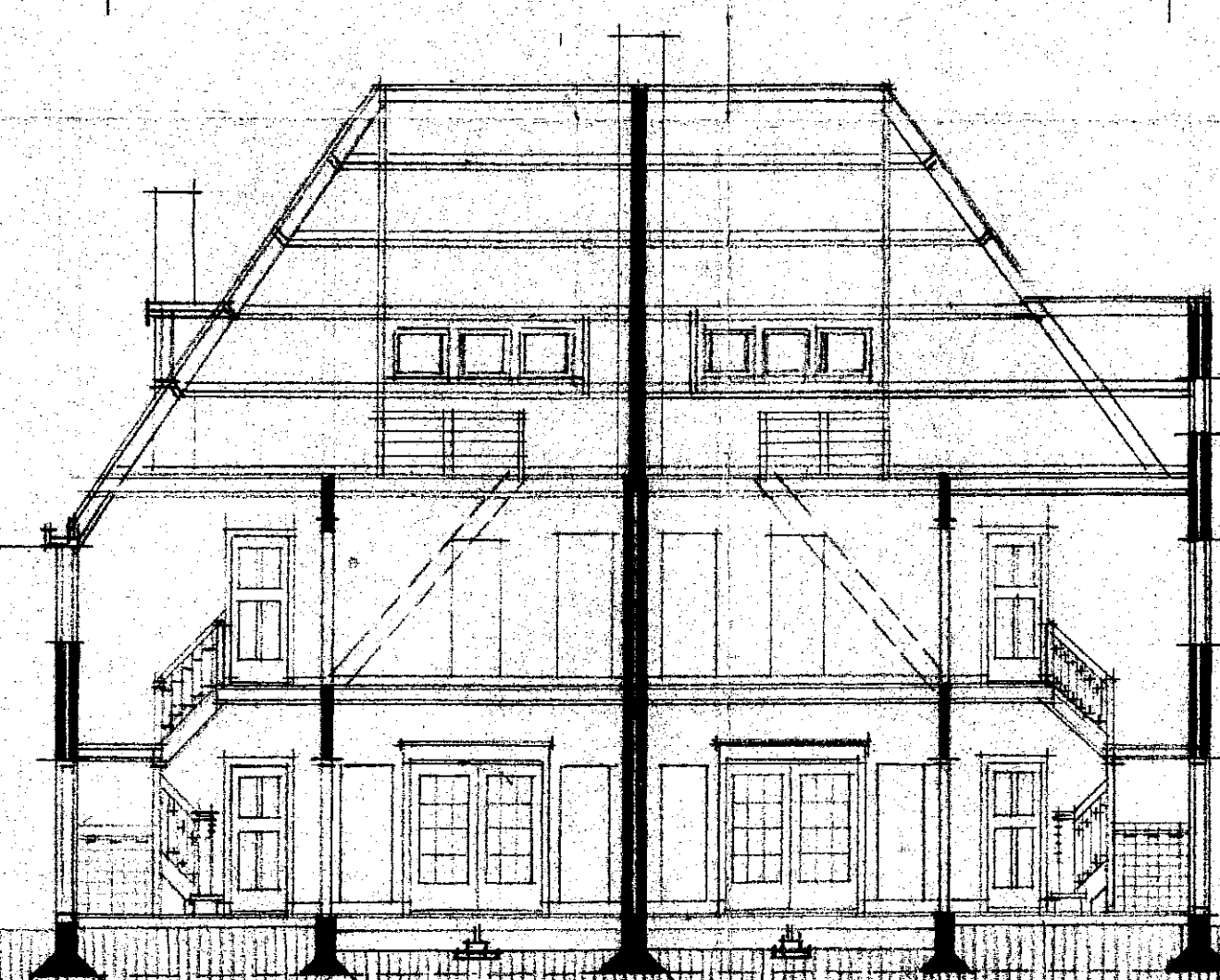
DOORSNEDEN A-B
