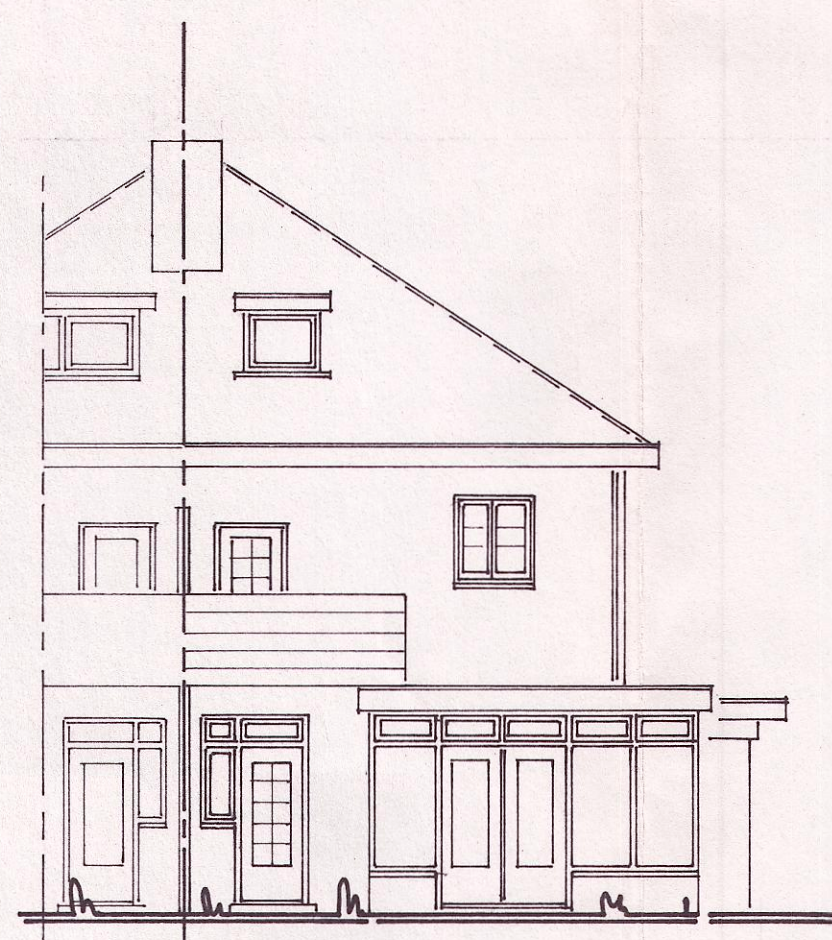
achtergevel bestaand
