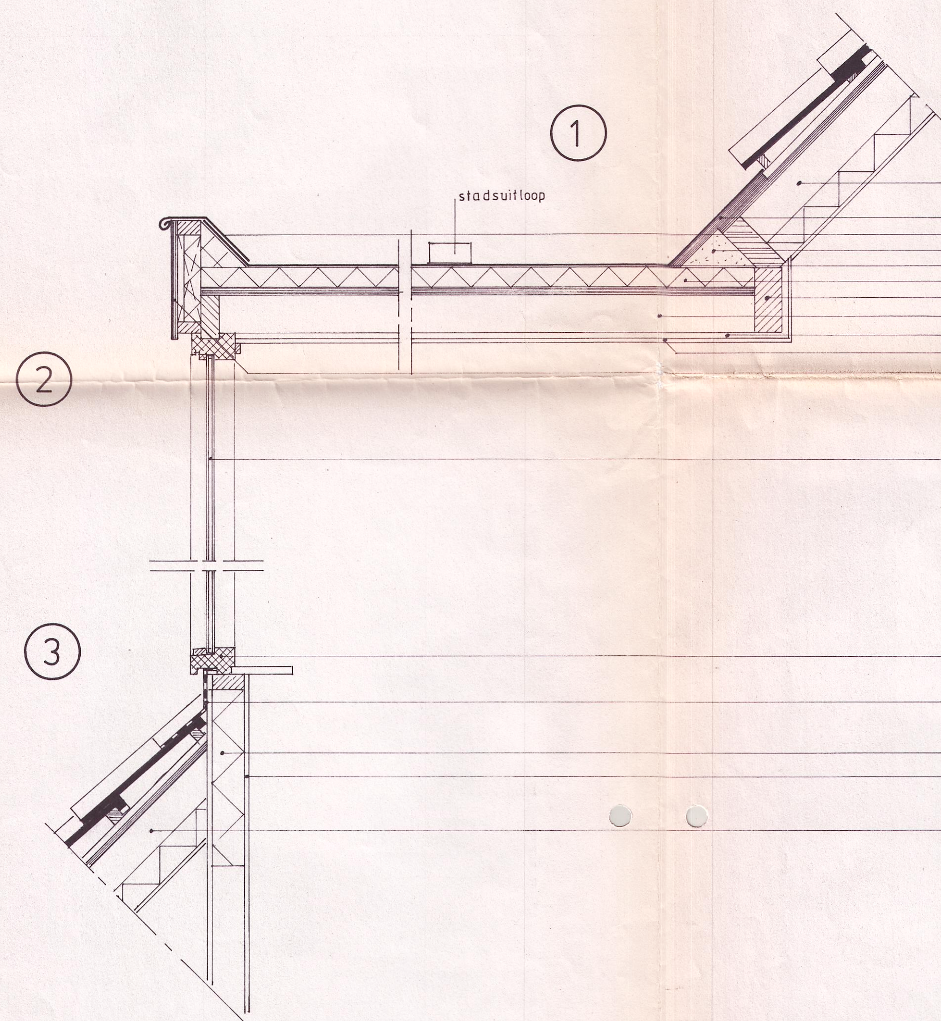
principe - details
