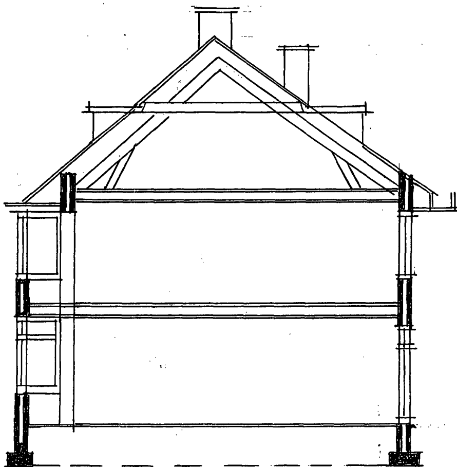
DOORSNEDE
