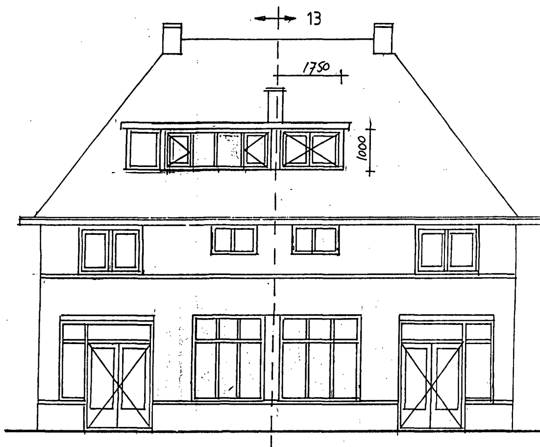
ACHTER GEVEL
