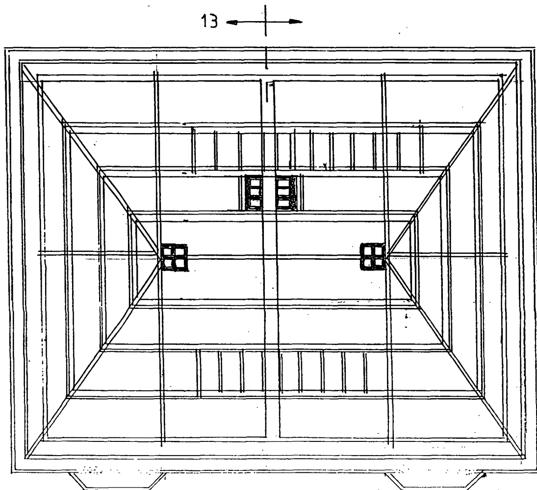
KAPPLAN
