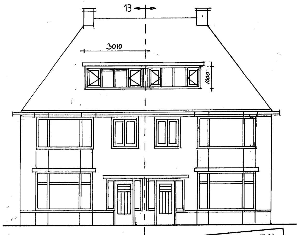
VOOR GEVEL
