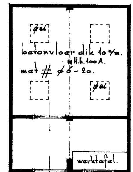
.plattegrond.
