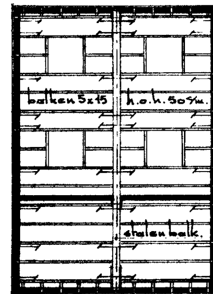
.plattbalklaag.
