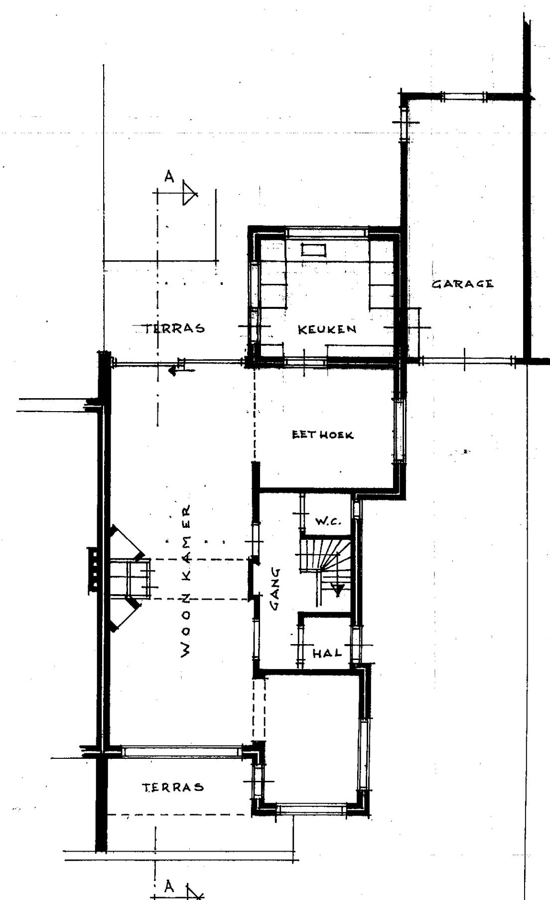
BEGANE GROND
