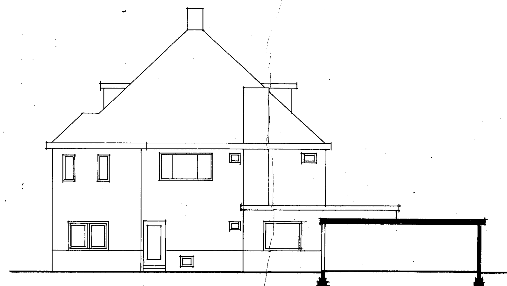
ZIJGEVEL
