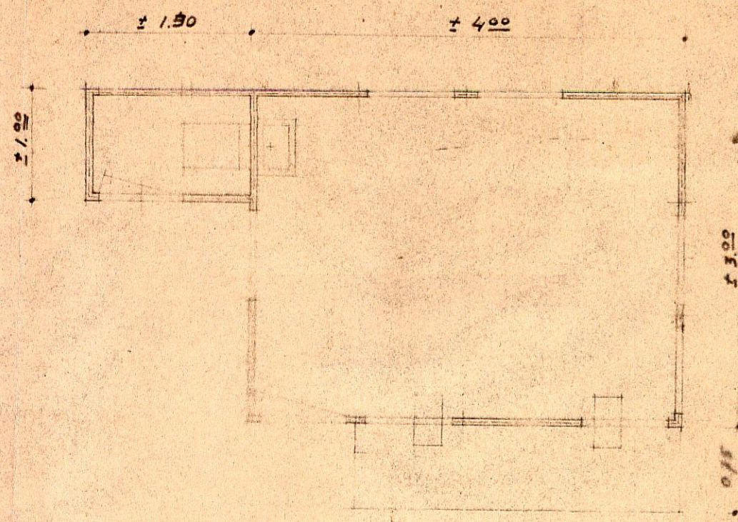
PLATTE GROND.
