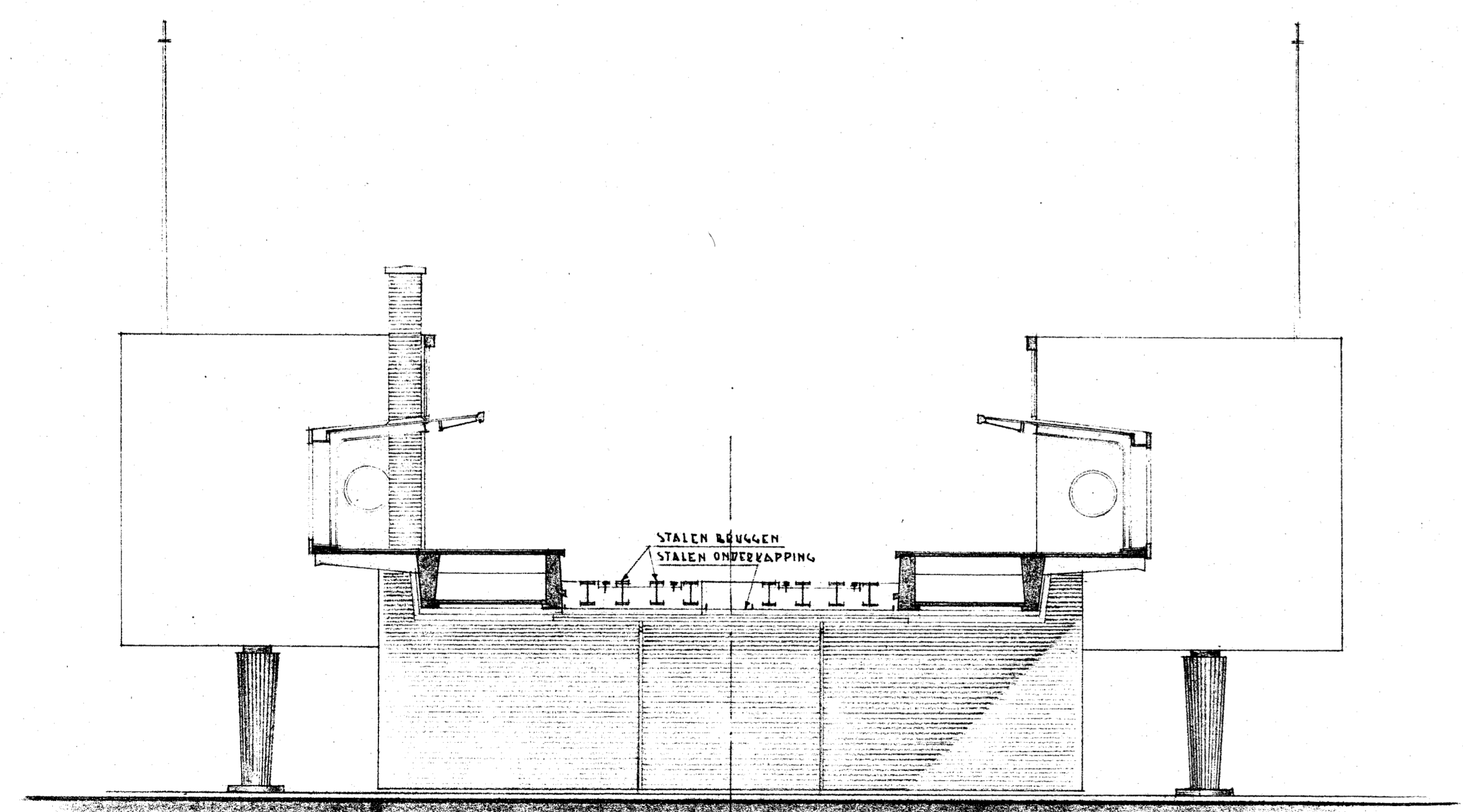
NOORDZIJDE HALTEGEBOUW.
