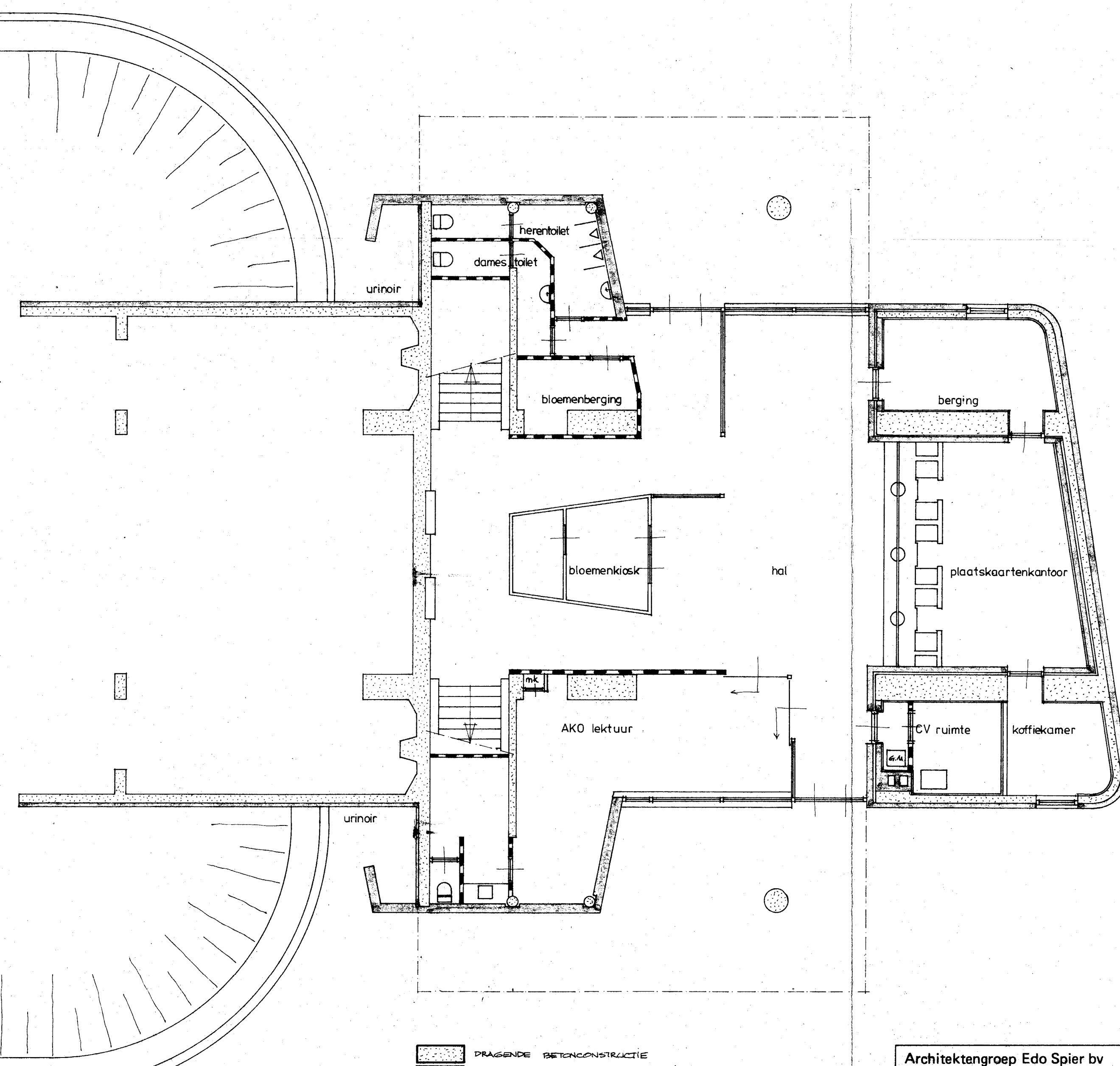
NIEUWE TOESTAND / PLATTEGROND EN ZUIDGEVEL
