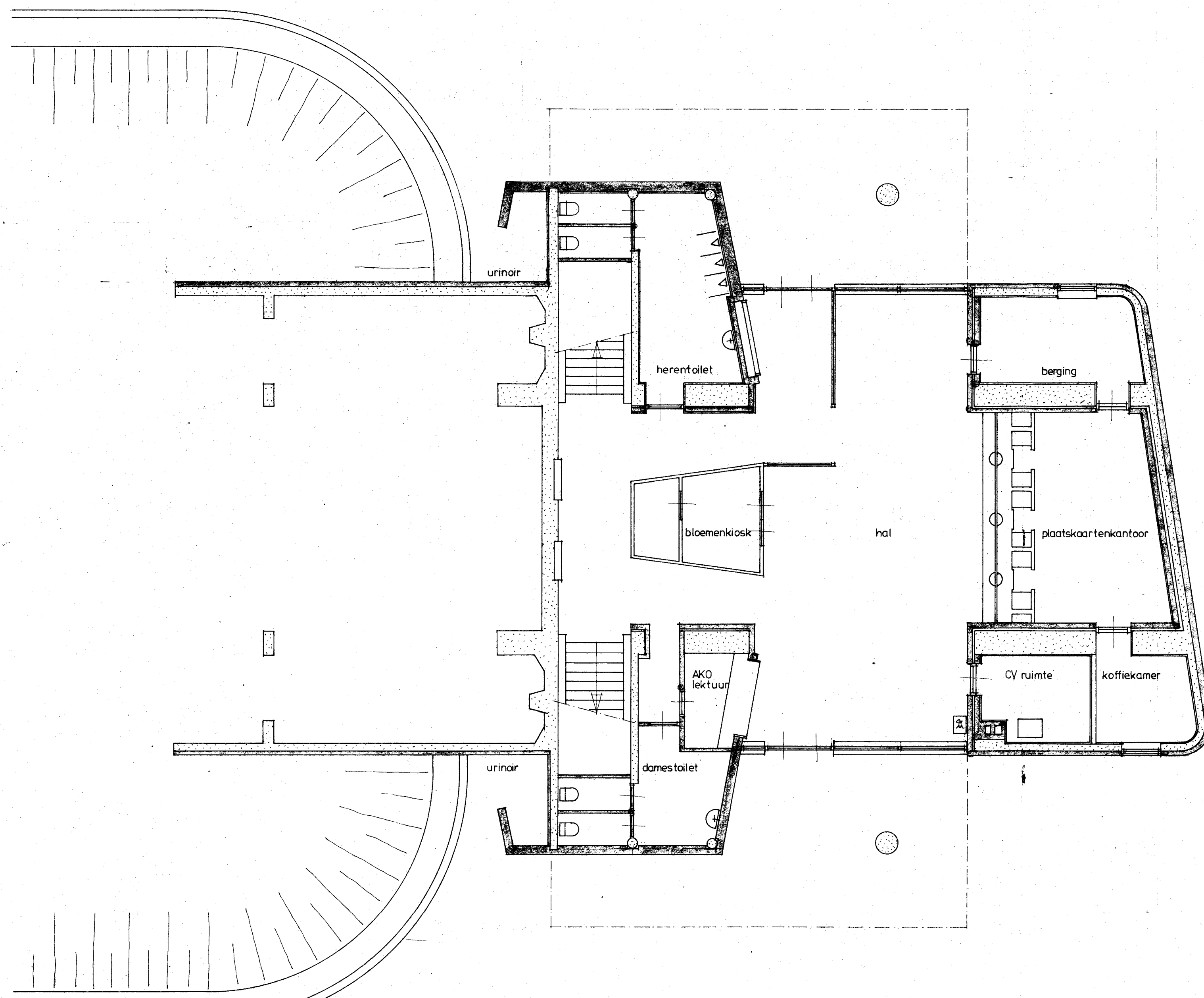
BESTAANDE TOESTAND / PLATTEGROND EN ZUIDGEVEL
