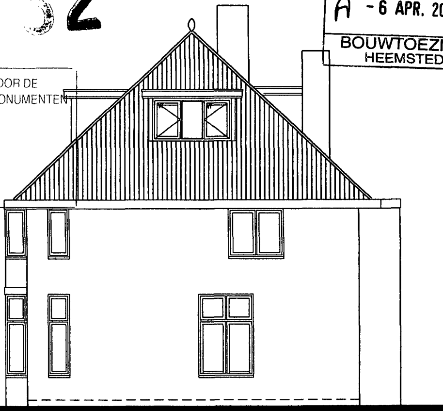
ZIJGEVEL
