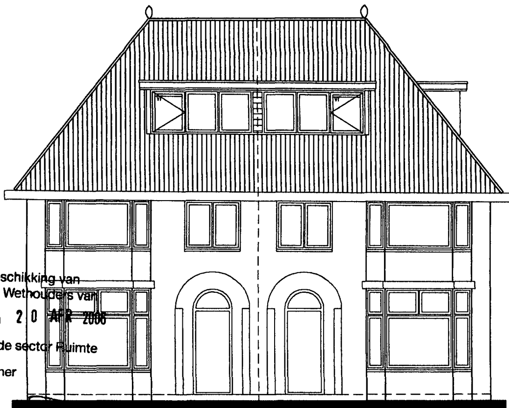
VOORGEVEL
