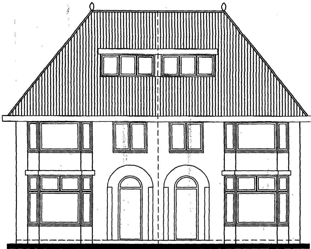
VOORGEVEL
