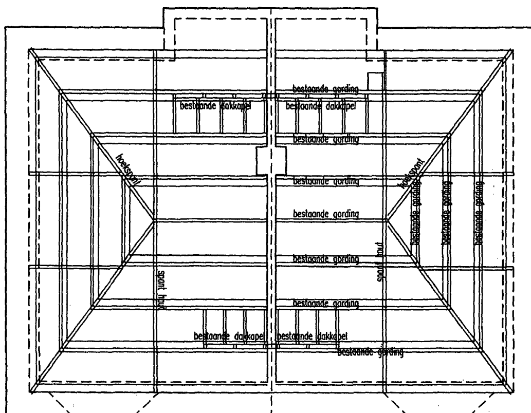
KAPCONSTRUCTIE
