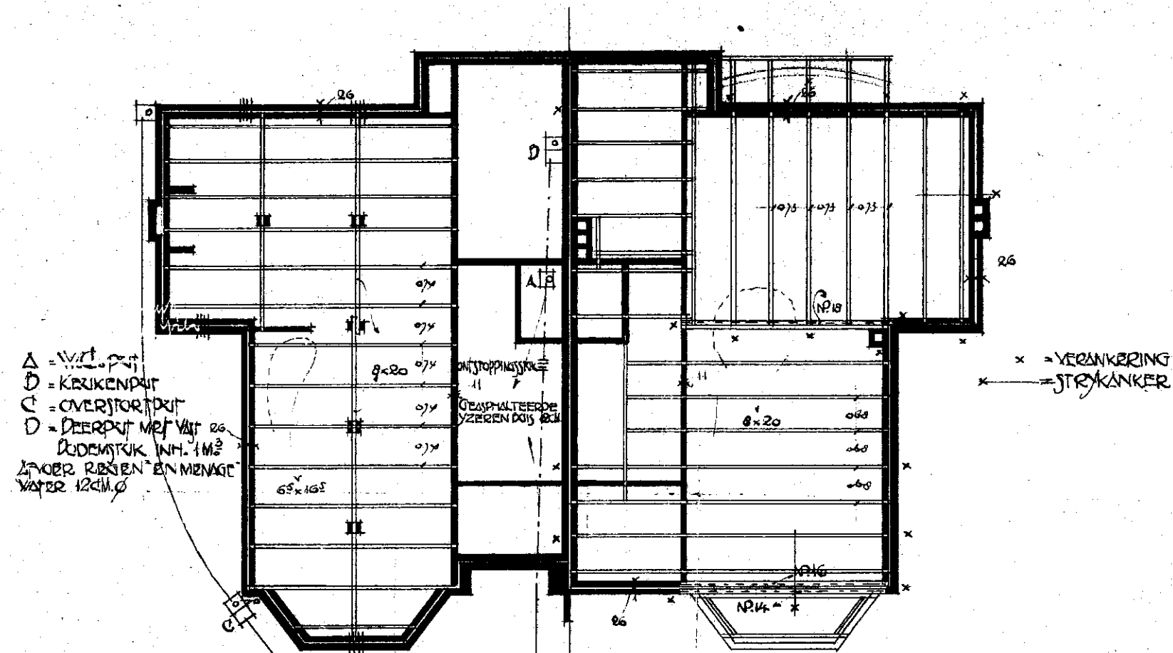
KEUKENLAAG
