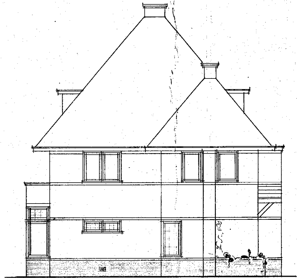
ZIJGEVEL
