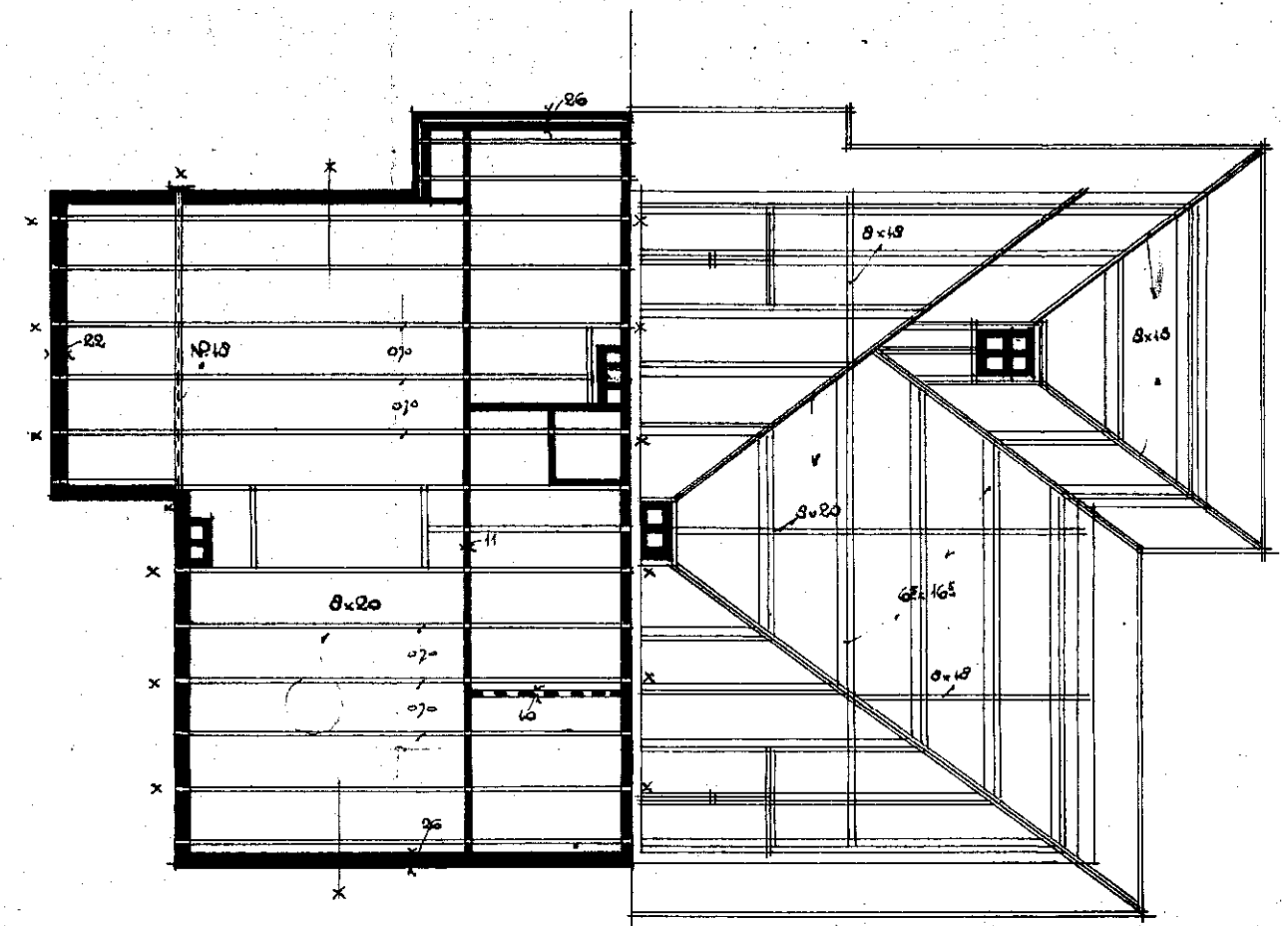
2 DE DALKLAAG
