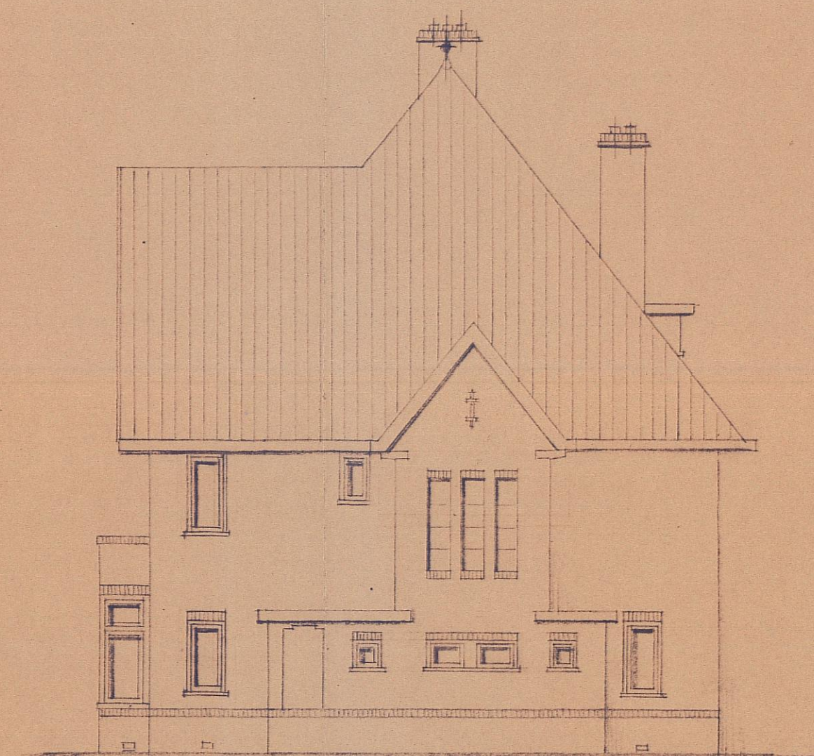
RECHTERGEVEL
