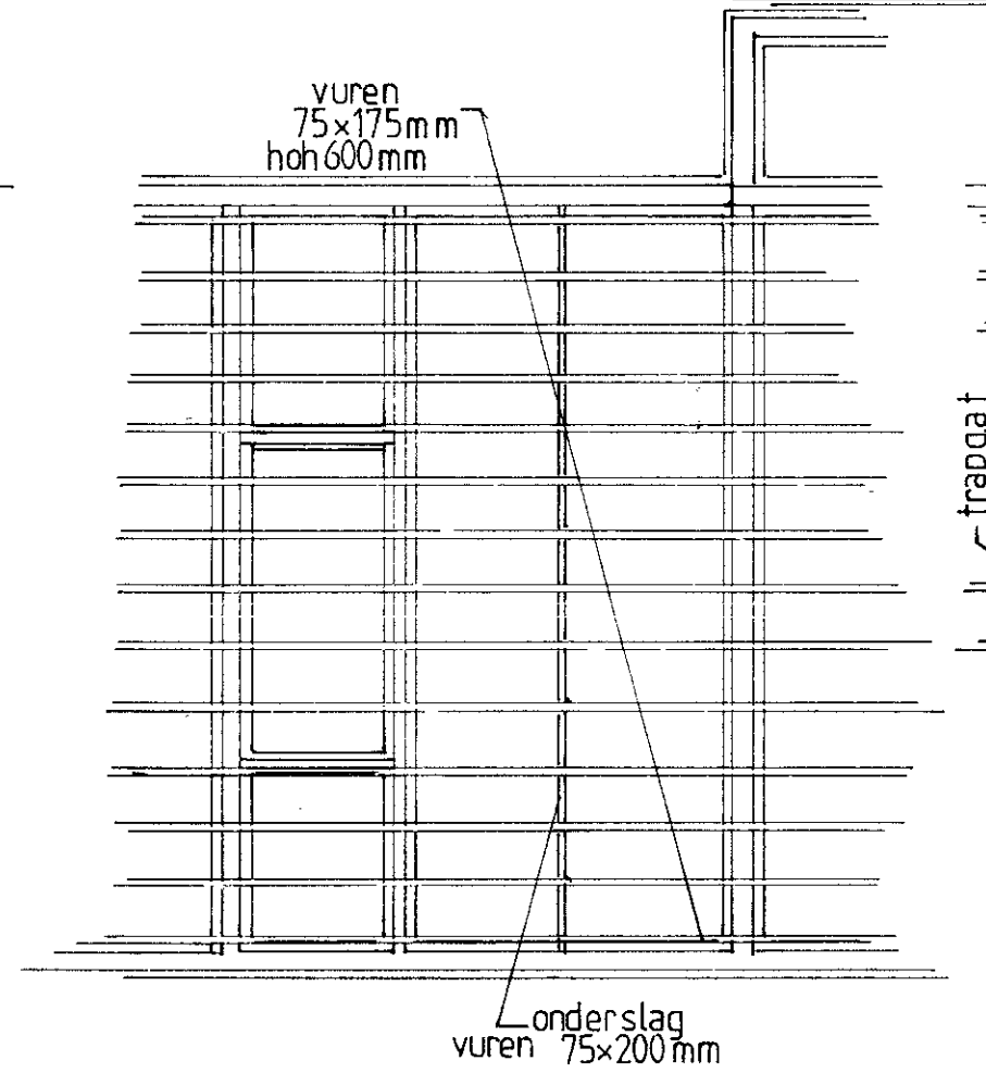
FUNDERING + VLOERBALKLAAG (blijft ongewijzigd)
