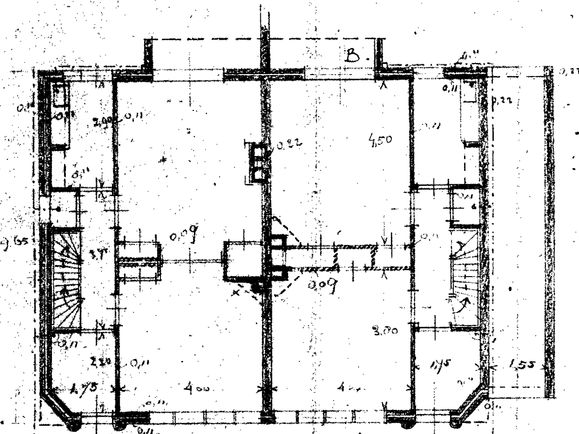
BEGINDE GROND
