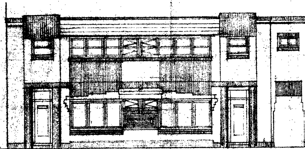
VOORGAVEL
