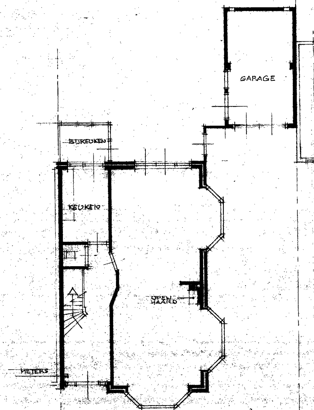
BEGANEGROND BESTAAND
