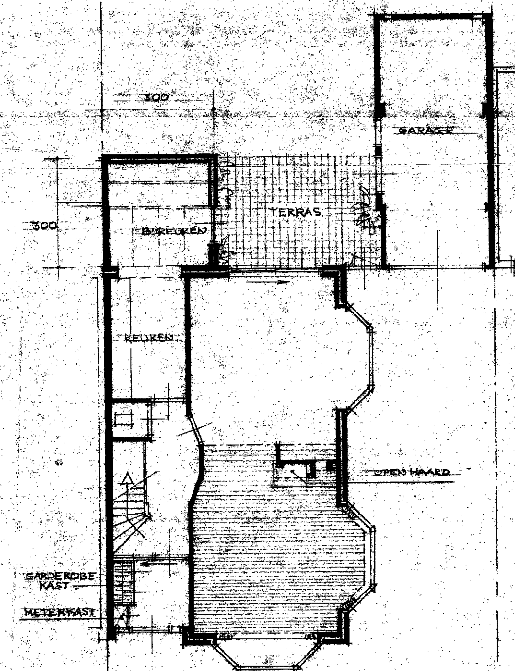
BEGANEGROND NIEUW
