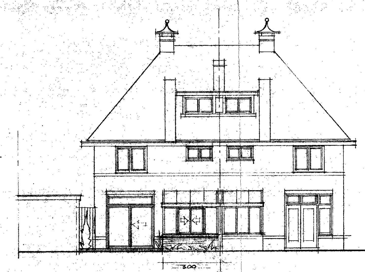
ACHTERGEVEL NIEUW
