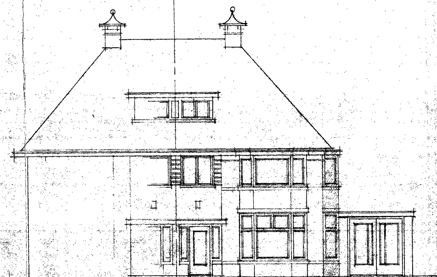
VOORGEVEL BESTAAND
