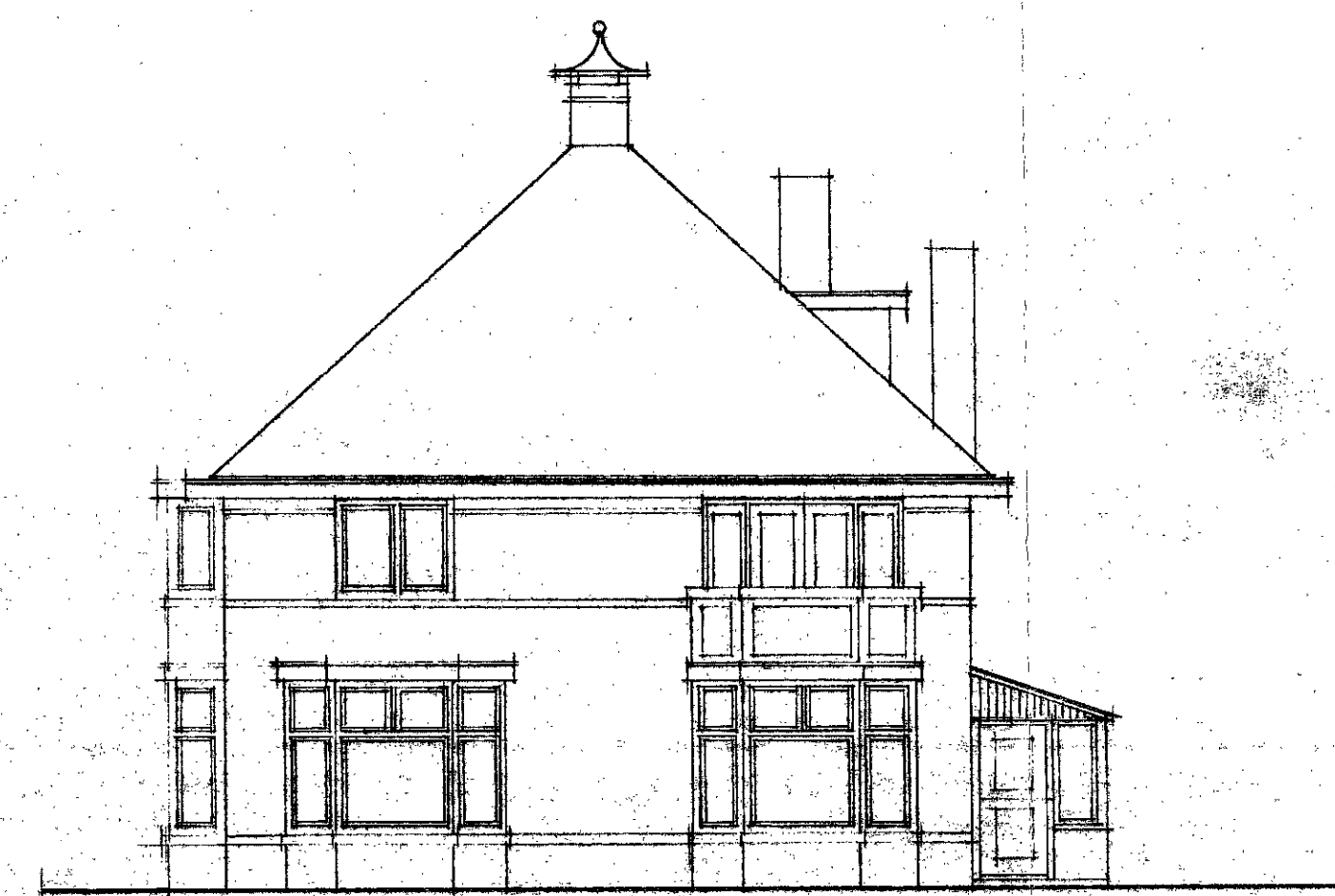
ZIJGEVEL BESTAAND
