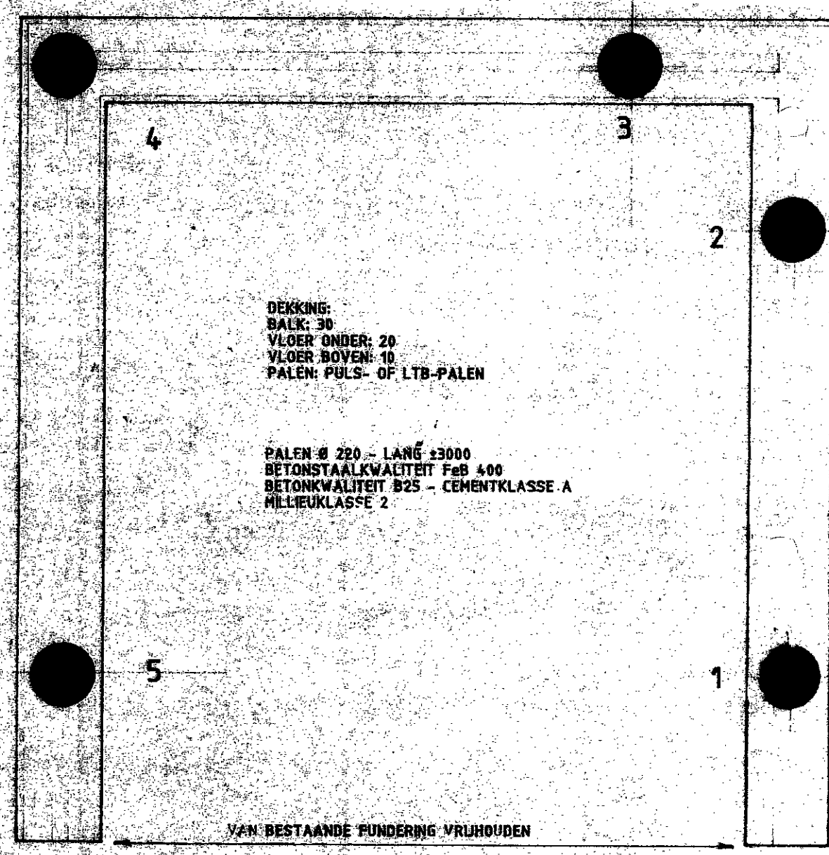
BEGANE GROND bestaande toestand
