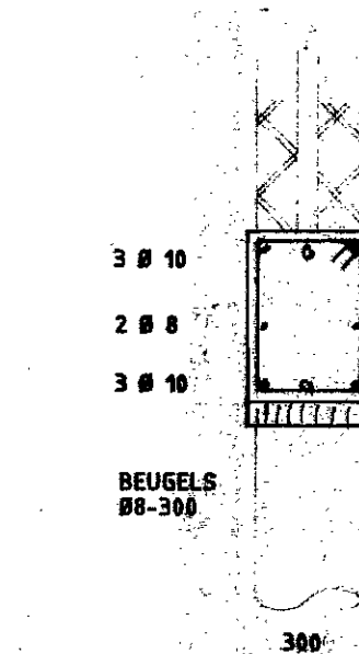
DOORSNEDE FUNDERINGSBALK
