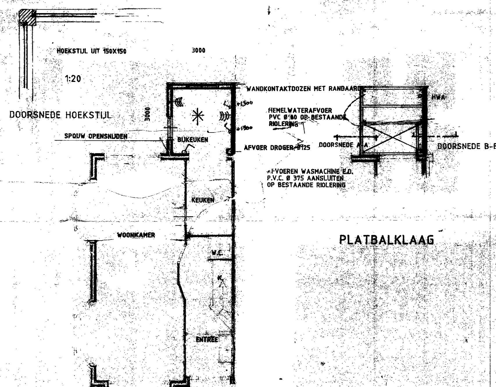
BEGANE GROND nieuwe toestand
