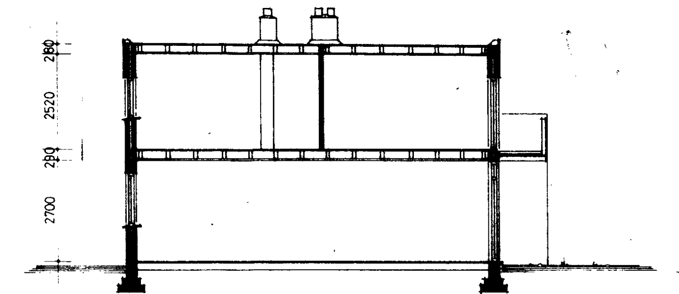
doorsnede A-A
