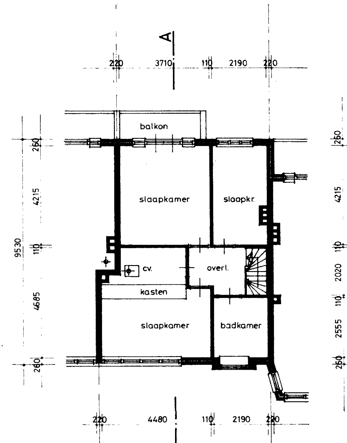
1e verdieping
